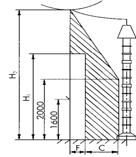
Şekil-7 Yere konulan ve geçitli normal çiti bulunan aygıtlarda koruma alanı
