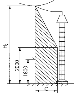
Şekil-6 Yere konulan ve geçersiz normal çiti bulunan aygıtlarda koruma alanı
