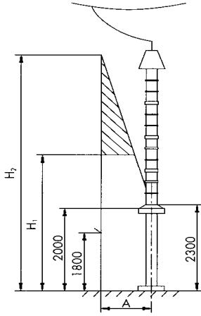
Şekil-5 Dayanak (mesnet) üzerindeki aygıtlarda koruma alanı
