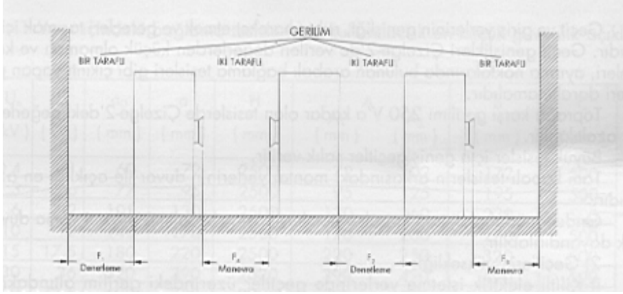
Şekil-1 Hücre cephelerinin tel kafes kapı ve dolu duvar olması durumunda geçit genişlikleri
