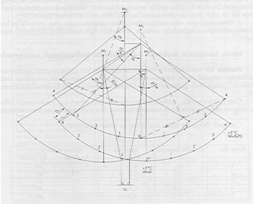
Şekil-8 İletken salınım diyagramı
