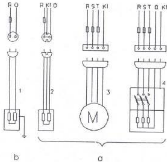
Şekil 8- Toprak teması akımının devresini su borusu şebekesi üzerinden kapadığı koruma topraklaması biçimleri
