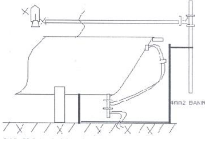
Şekil -22 Potansiyel dengeleminin yapılışı
