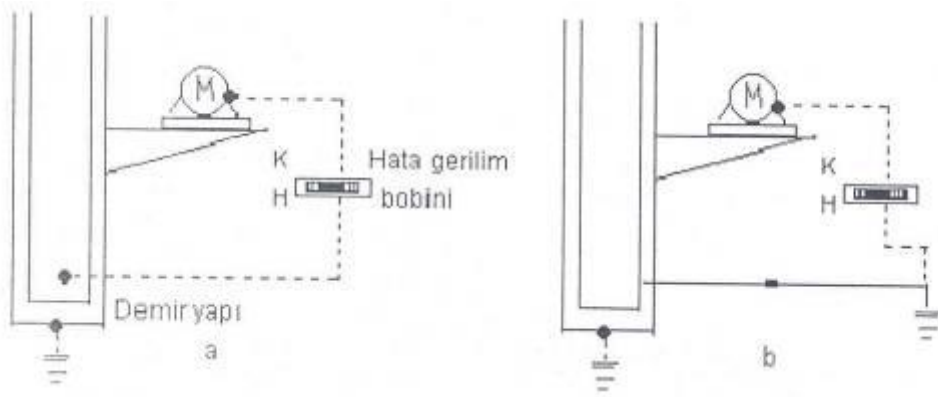
Şekil - 15 Hata gerilimi bobininin bağlanması
